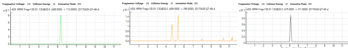
图 B.4 硫代艾地那非
