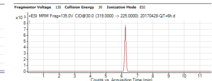
图 B.42 酚酞
