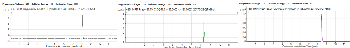
图 B.1 利血平
